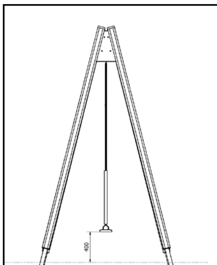
Kumilautaisuimen maavara on 400 mm.
