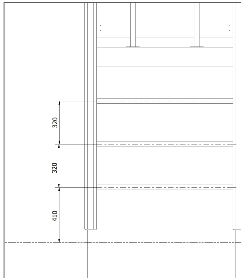
Kiipeilytankojen etäisyys toisistaan ja etäisyys maasta
