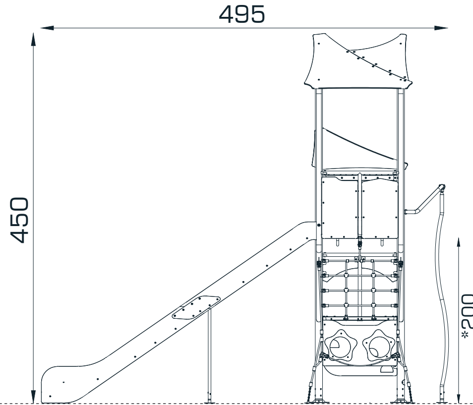
ÖN GÖRÜNÜŞ / FRONT VIEW
